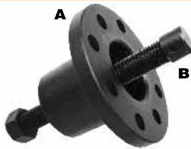
CR 139 A Ferramenta avulsa para uso c/ CR 80 ou com CR 139-B
